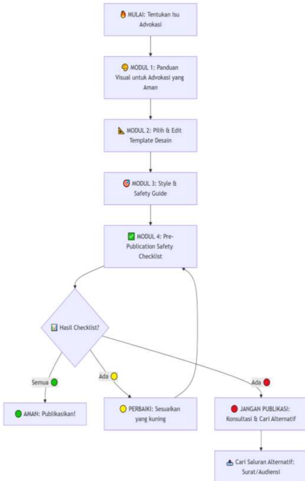
Gambar 2. Alur Kerja
