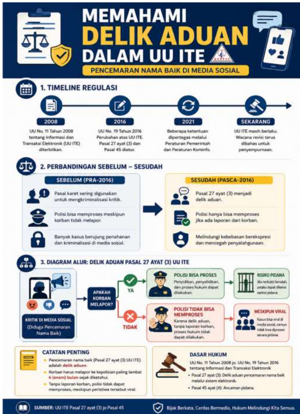
Gambar 7. Contoh Infografik
